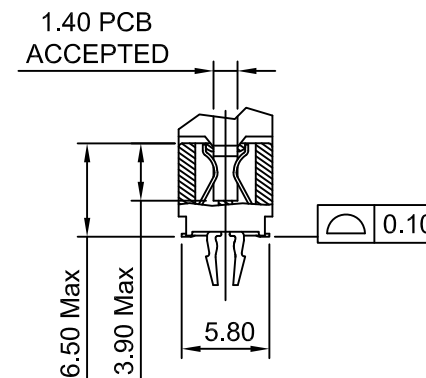
SEC: A-A SCALE 2:1
