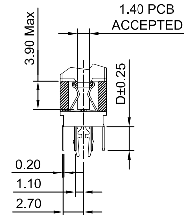
SECTION A-A SCALE 2:1
