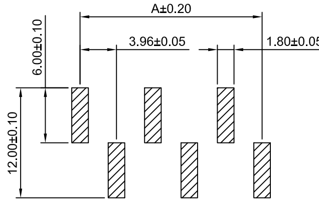
P.C.B LAYOUT
