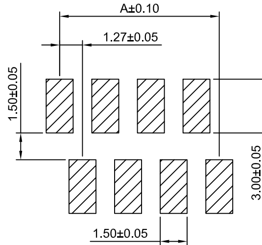
P.C.B LAYOUT
