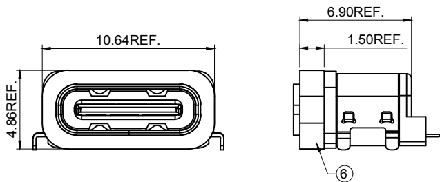
防水圈组装示意图
