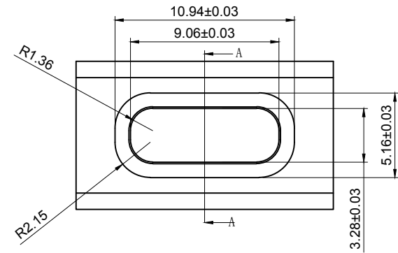
c 机壳开孔建议尺寸图
