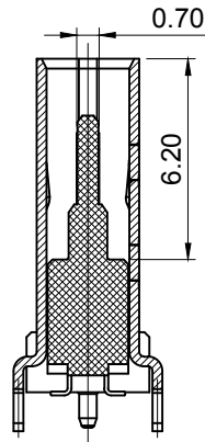
SECTION A-A SCALE 1:1
