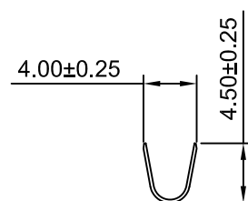
SEC:B-B
