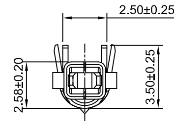
SEC:A-A
