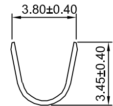
SEC:B-B
