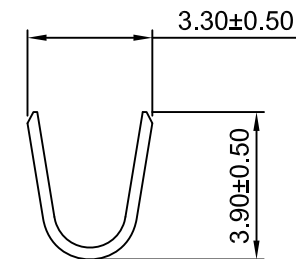
SEC:B-B
