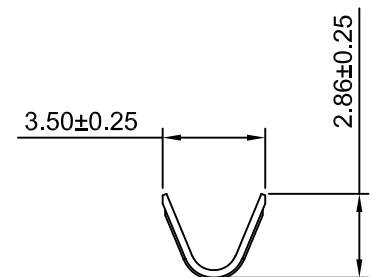
SEC:B-B
