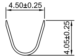
SEC:A-A
