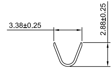
SEC:B-B
