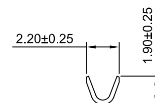
SEC: A-A
