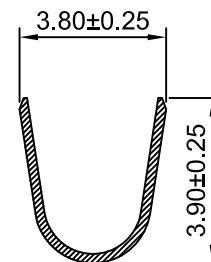
SEC:B-B
