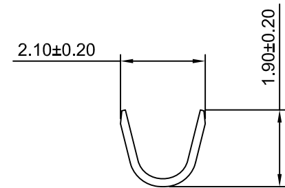
SEC:A-A
