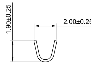
SEC:B-B
