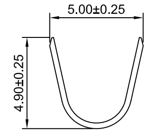
SEC:A-A
