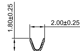
SEC:B-B
