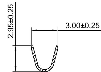
SEC:A-A
