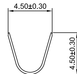
SEC:A-A
