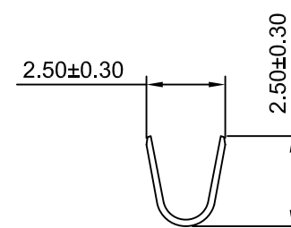
SEC:B-B
