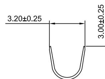
SEC:A-A
