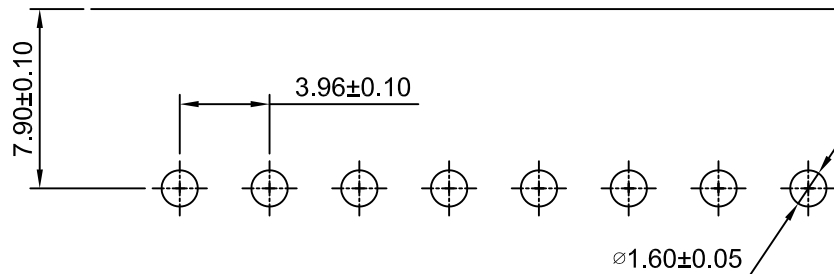
P.C.B LAYOUT
