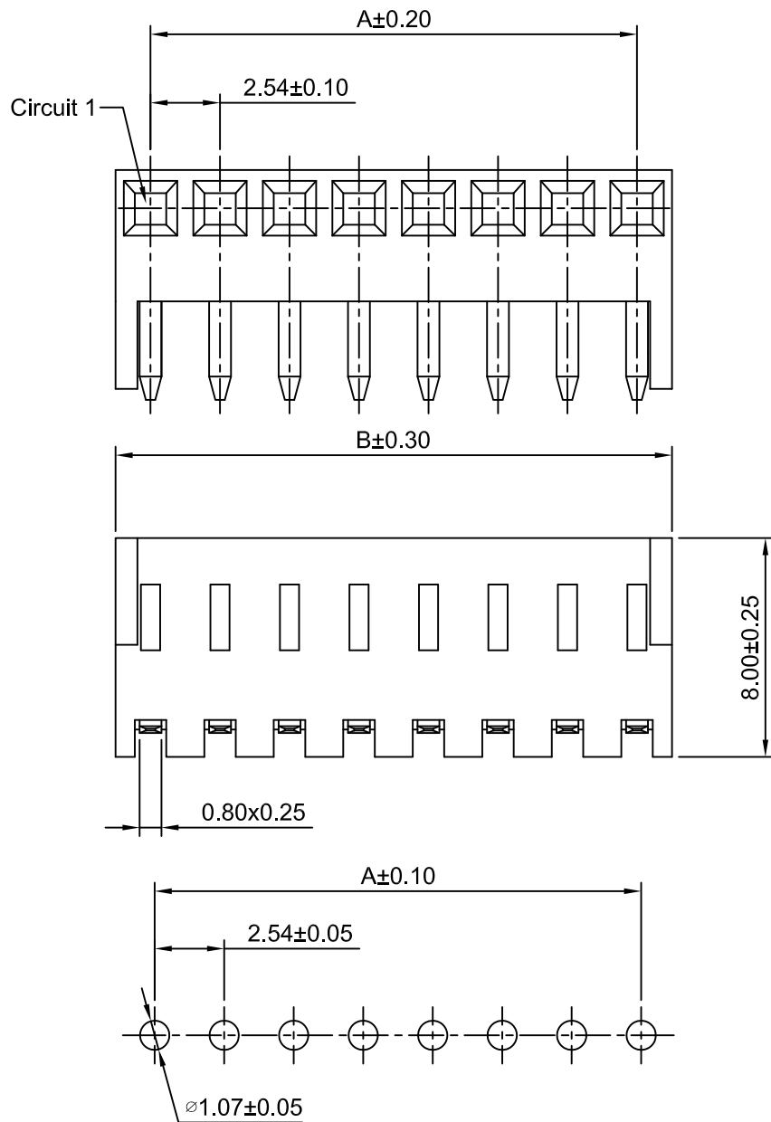
P.C.B LAYOUT
