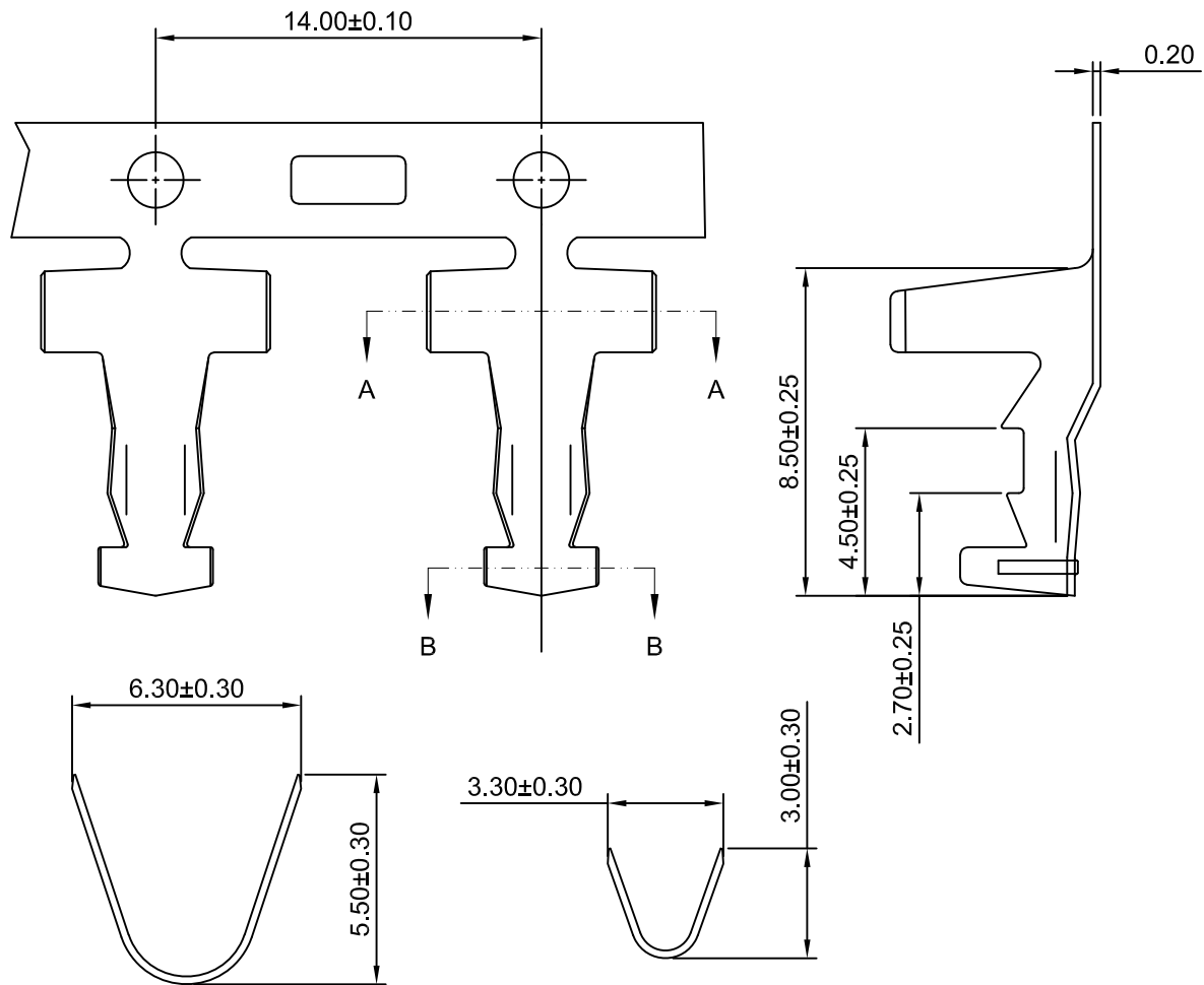
SEC:B-B
