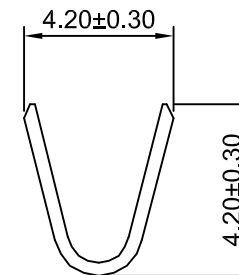
SEC: B-B
