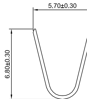
SEC: A-A
