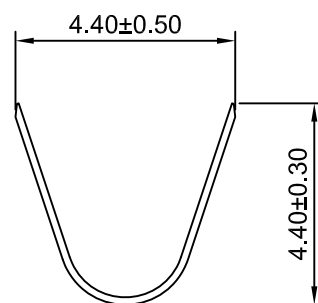
SEC:A-A
