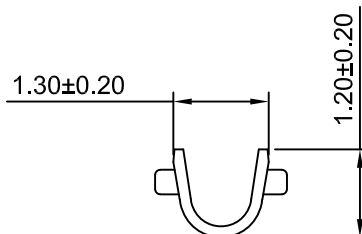
SEC: B-B
