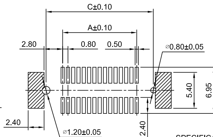
P.C.B LAYOUT
