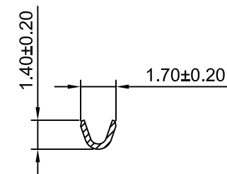
SEC:A-A
