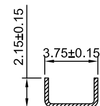
SEC:B-B
