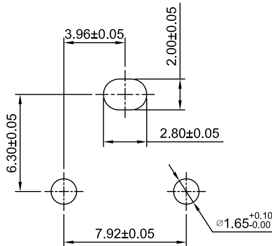
P.C.B LAYOUT
