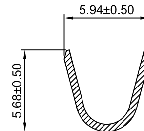
SEC:A-A
