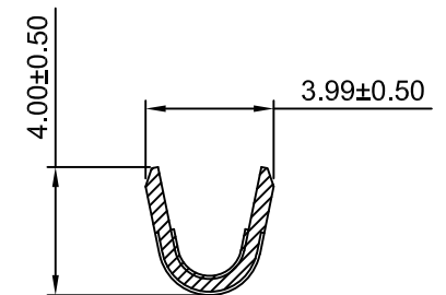
SEC:B-B
