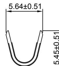
SEC:A-A
