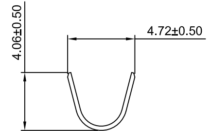
SEC:A-A
