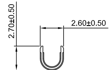
SEC:B-B
