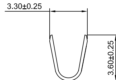
SEC:A-A
