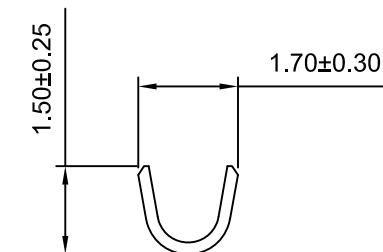
SEC:B-B
