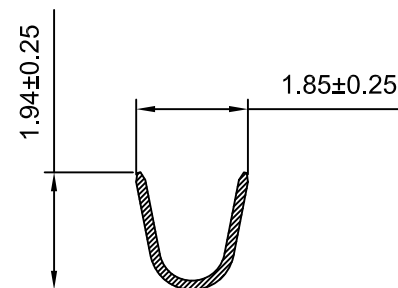
SEC:A-A
