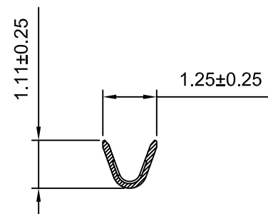
SEC:B-B
