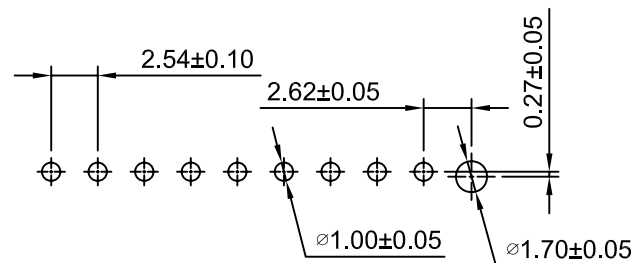
P.C.B LAYOUT
