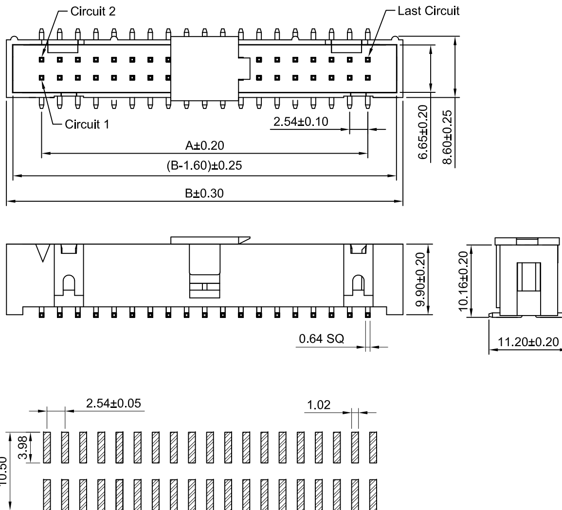
P.C.B LAYOUT
