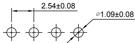
P.C.B LAYOUT
