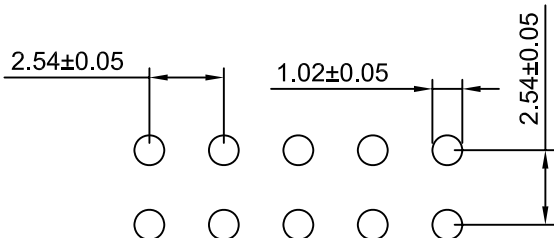
P.C.B LAYOUT
