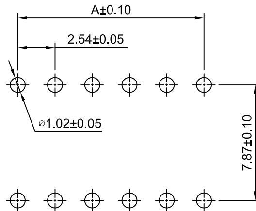
P.C.B LAYOUT
