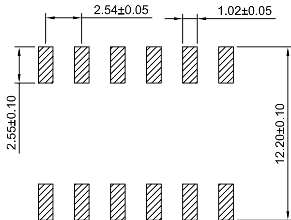
P.C.B LAYOUT
