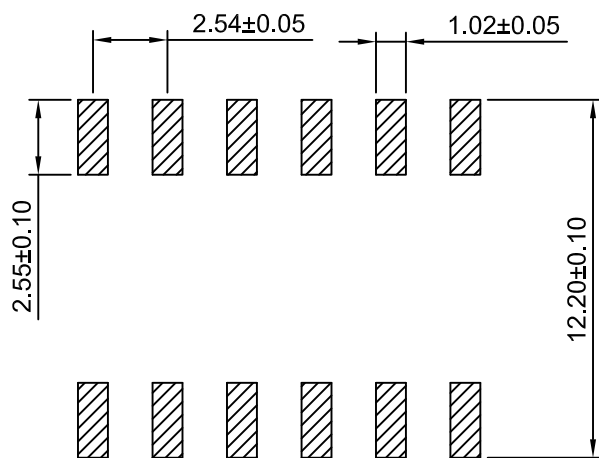
P.C.B LAYOUT
