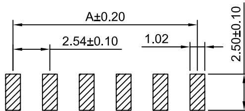
P.B.C LAYOUT
