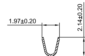
SEC:B-B
