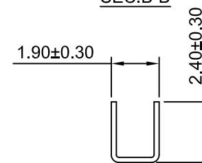
SEC:B-B
