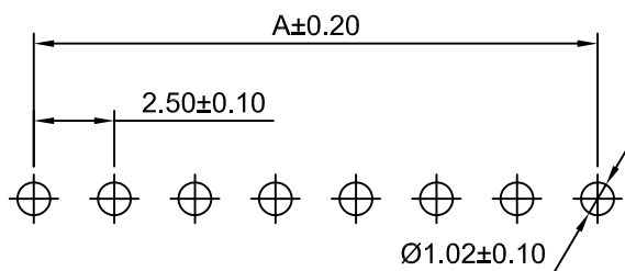
P.C.B LAYOUT
