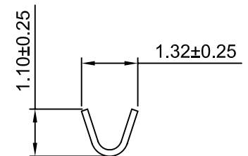
SEC:B-B
