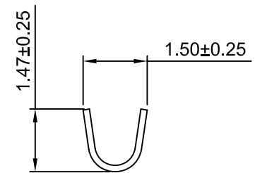
SEC:A-A
